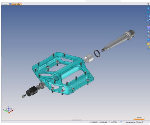
Konstruktion und Erstellung von 3D-Modellen der MTB-Pedalen.
