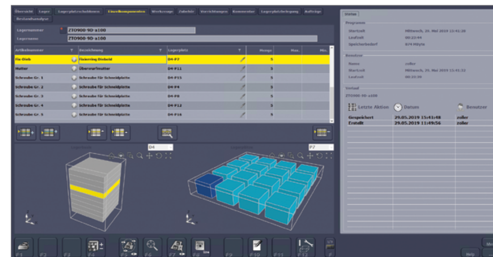
Softwaremodul Lagerverwaltung
